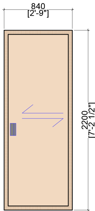
D5 SLIDING DOOR
